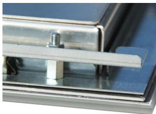
Detail Klemme, Bolzen und Federlaschenverbindung
