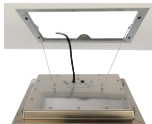
Mit Aufnahmerahmen
